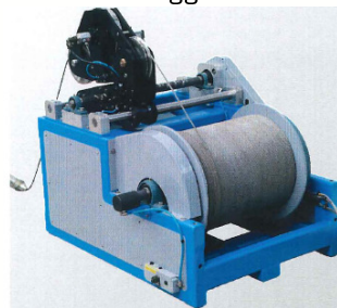
3000m級Winch
