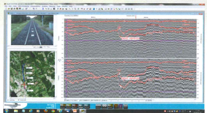
鉄道への適用例(GPR,線路画像)
