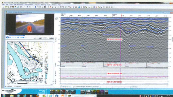
道路への適用例(GPR,FWD,IRI)
